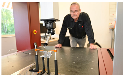
Björn mäter upp en komplex detalj som serietillverkas med hög teknisk precision – och "oöverträffad snabbhet".
