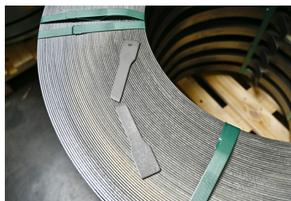
Testad – till bristningsgränsen. GA Industri ligger steget före och erbjuder sina kunder tester av plåtens mekaniska egenskaper.
