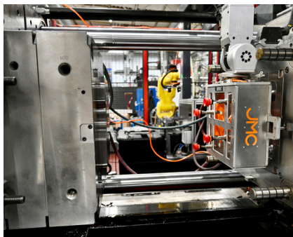
Vissa av detaljerna körs i högre volymer i en hel-automatisk produktionscell för ingjutning av bussningar.
